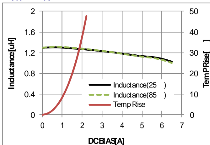
・AMC0312-1R5C
