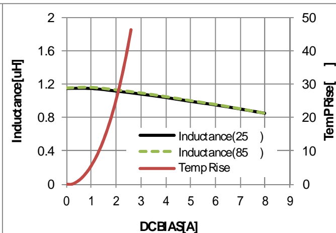
・AMC0312-1R2C
