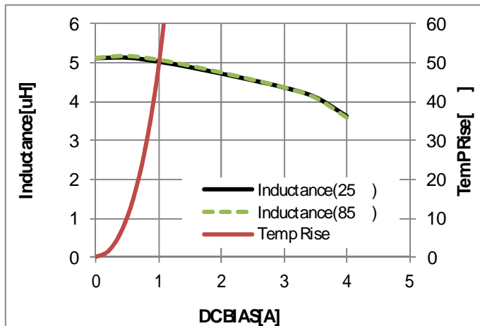
・AMC0312-5R6
