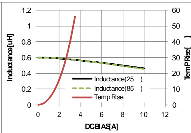
・AMC0312-R68C
