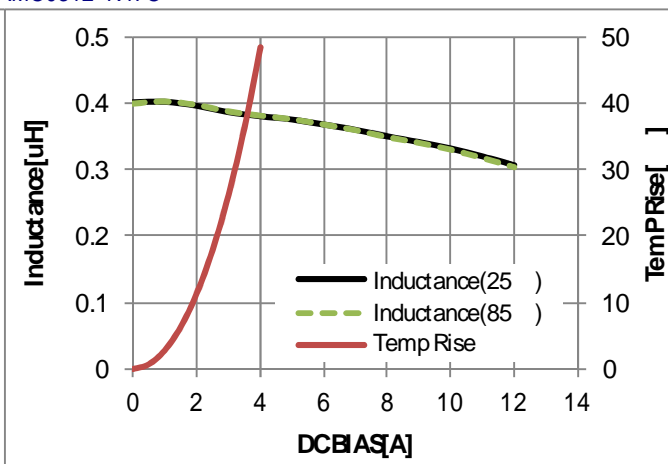
・AMC0312-R47C
