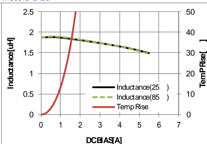
・AMC0312-2R2C
